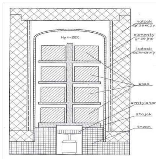
Ryc. 1. Schemat pieca kołpakowego
