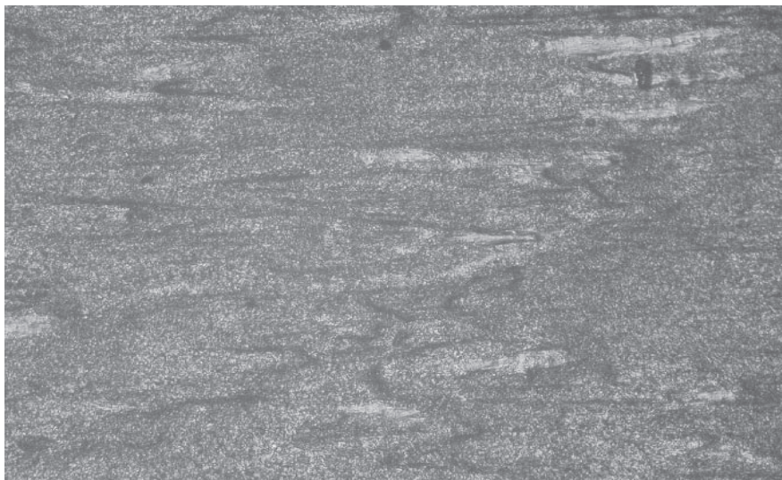
Ryc. 5. Mikrostruktura taśmy z mosiądzu M70 wyżarzanej w dolnej strefie starego pieca kołpakowego
