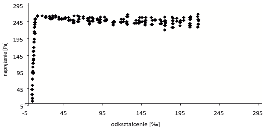
Ryc. 8. Wykres naprężenia od odkształcenia dla 10% zawiesiny korundu w polu elektrycznym o natężeniu 2 kV/mm
