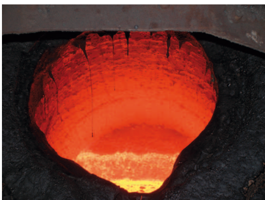
Ryc. 2. Kadź żeliwiakowa wymurowana nowymi wyrobami wysokoglinowymi modyfikowanymi SiC w trakcie eksploatacji (A) i po wystudzeniu (B)
