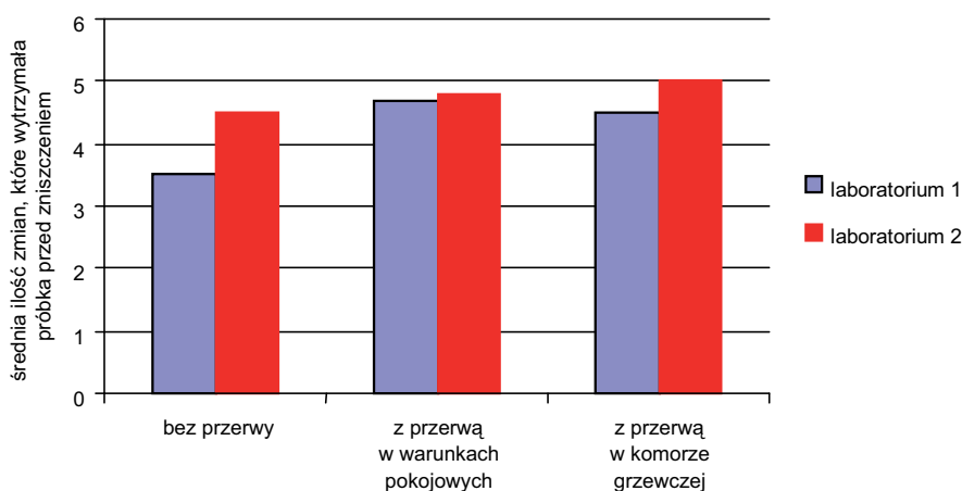
Ryc. 5. Odporność na wstrząsy cieplne dla próbek walcowych ogrzewanych do temperatury 950°C, a następnie chłodzonych wodą
