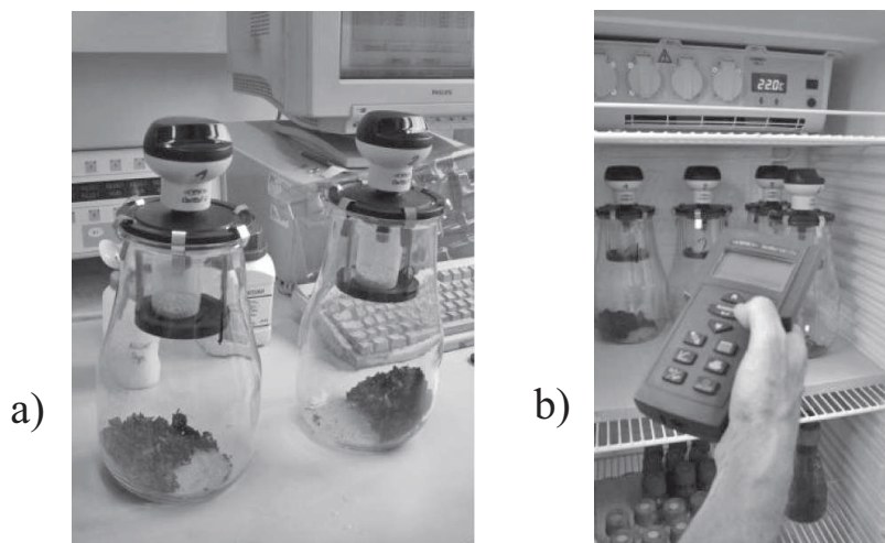
Ryc. 3. Zestaw OxiTop: a) naczynia z próbką, b) naczynia umieszczone w szafie termostaticznej wraz z kontrolerem
