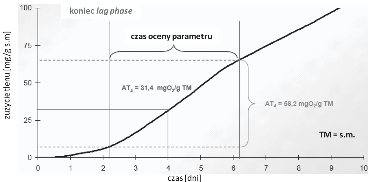
Ryc. 2. Przykładowy wykres zużycia tlenu w czasie z zaznaczoną fazą przygotowawczą
