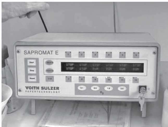
Ryc. 1. Zestawy SAPROMAT umieszczone w łaźni oraz jednostka sterująca dozowanie tlenu
