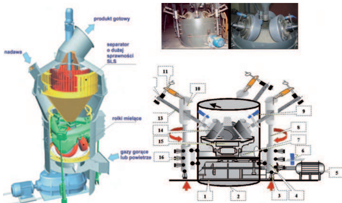
Ryc. 3. Schemat młyna firmy Pfeiffer i układu mielącego młyna rolkowo-misowego w skali półtechnicznej: 1 – przekładnia kąтова, 2 – obudowa, 3 – śruba regulacji pionowej, 4 – tuleja, 5 – silnik napędowy, 6 – czujnik obrotów, 7 – zgarniaki, 8 – wspornik rolki, 9 – czujnik obrotów rolki, 10 – element walcowy, 11 – czujnik tensometryczny, 12 – sprzęgło śrubowe, 13 – osie rolek, 14 – rolka, 15 – misa, 16 – śruby regulacji poziomej [14]
