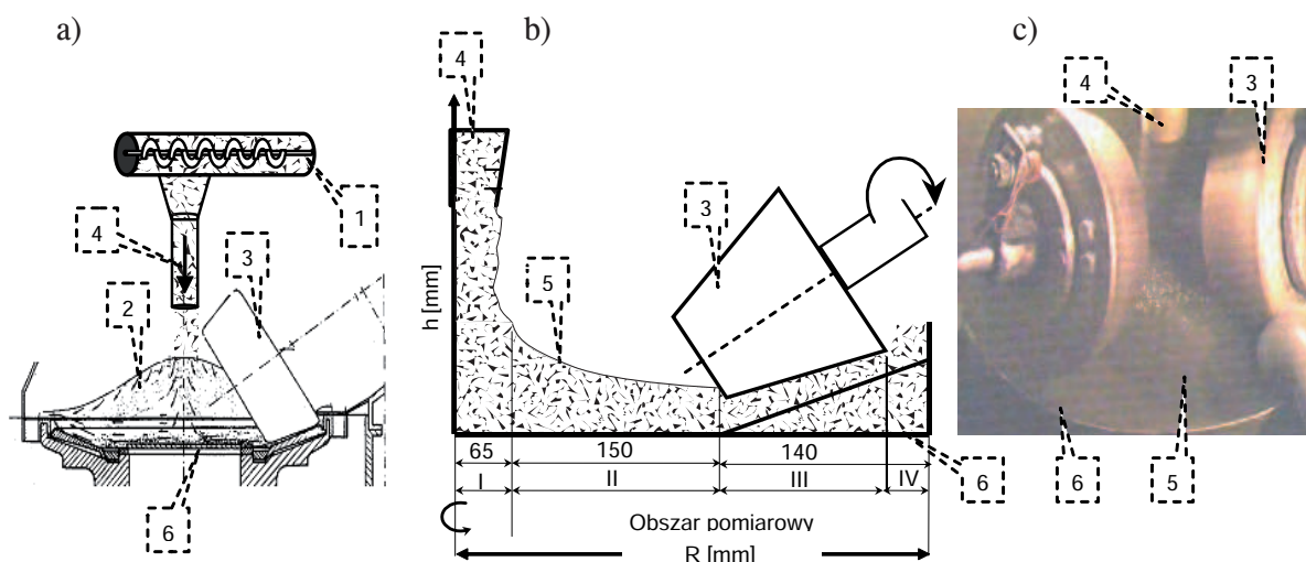
Ryc. 4: a) analizowany układ mielący , b) strefy pomiarowe, c) pracujący układ mielący: 1 – podajnik, 2 – warstwa mielniwa, 3 – rolka mieląca, 4 – rura zsygową, 5 – wysokość warstwy mielniwa na misie, 6 – tor mielenia
