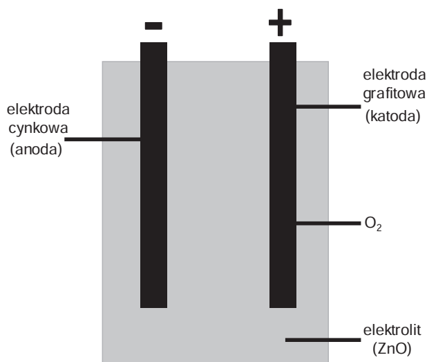
Ryc. 5. Schemat ogniw cynkowo-tlenowego
