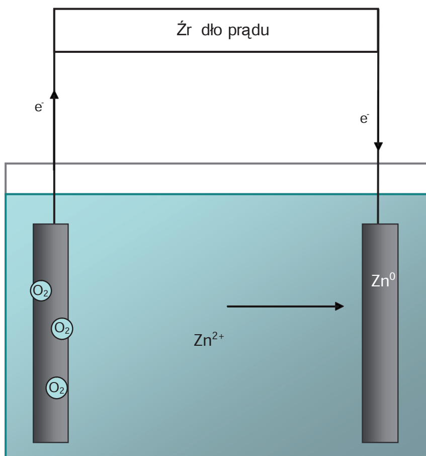
Ryc. 4. Schemat urządzenia do elektrolizy roztworu cynku
