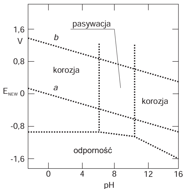
Ryc. 3. Diagram pourbaix dla cynku E^\circ w funkcji pH [8]
