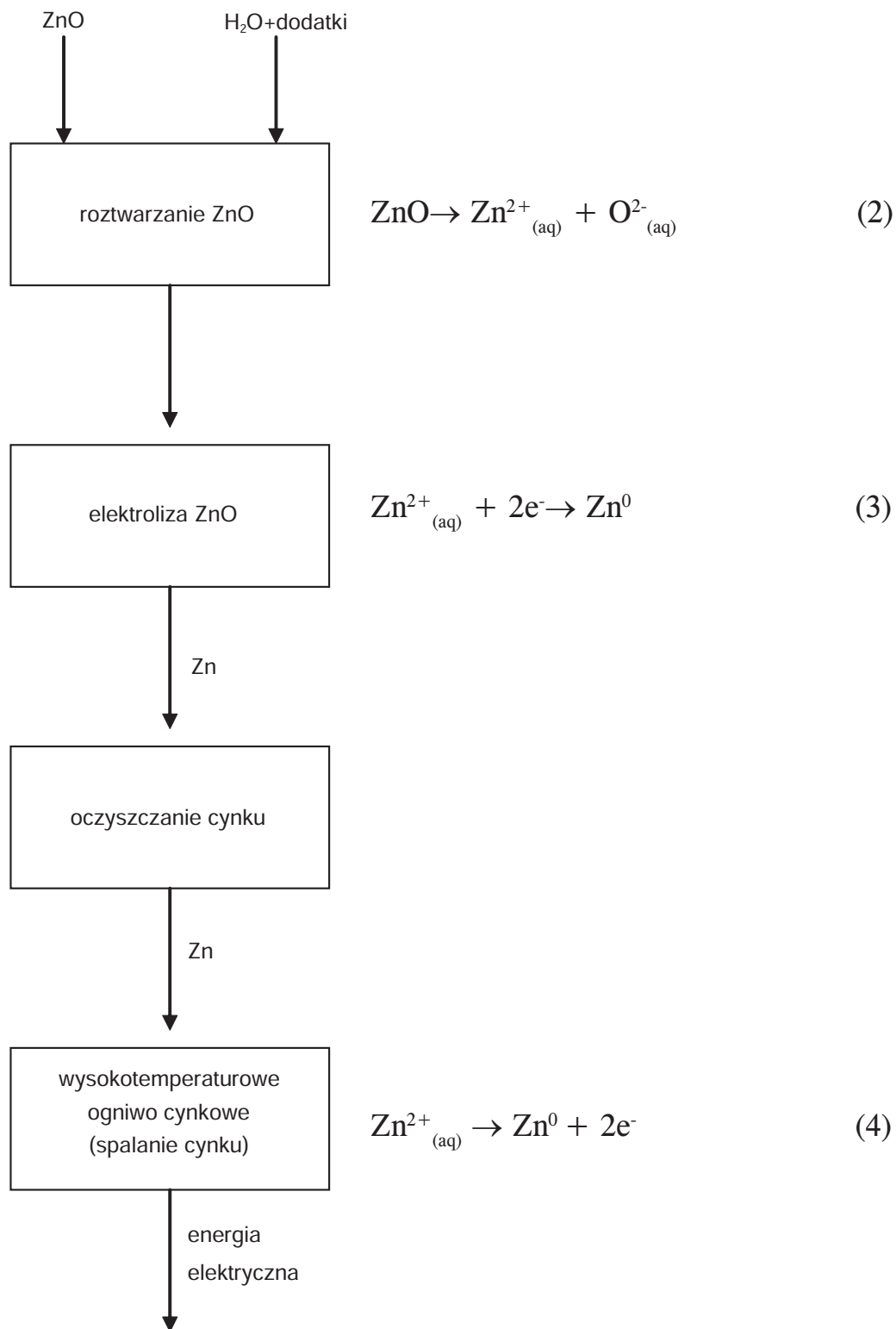
Ryc. 2. Schemat ciągu technologicznego magazynu energii
